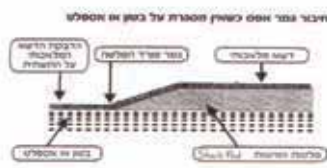
"דשא פלקס" בחתך מהצד
